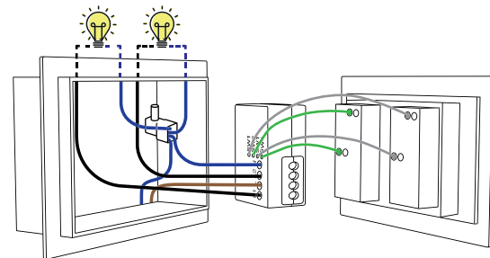
B. Collegamento di due interruttori;
