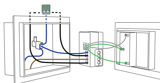
G. Collegamento commutatore (tapparella);
