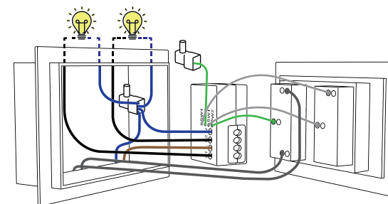
D. Collegamento di un deviatore e un interruttore;
