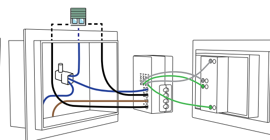
H. Collegamento doppio pulsante (tapparella);
