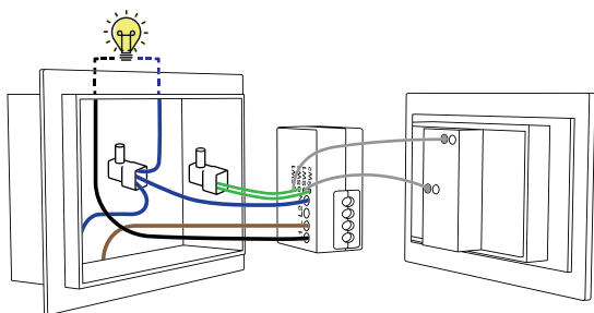
A. Collegamento di un interruttore;
