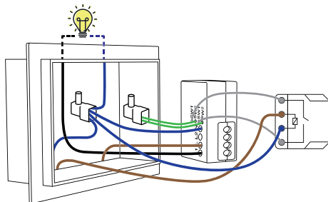
E. Collegamento di un relè;
