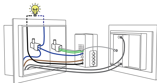
C. Collegamento di un deviatore;
